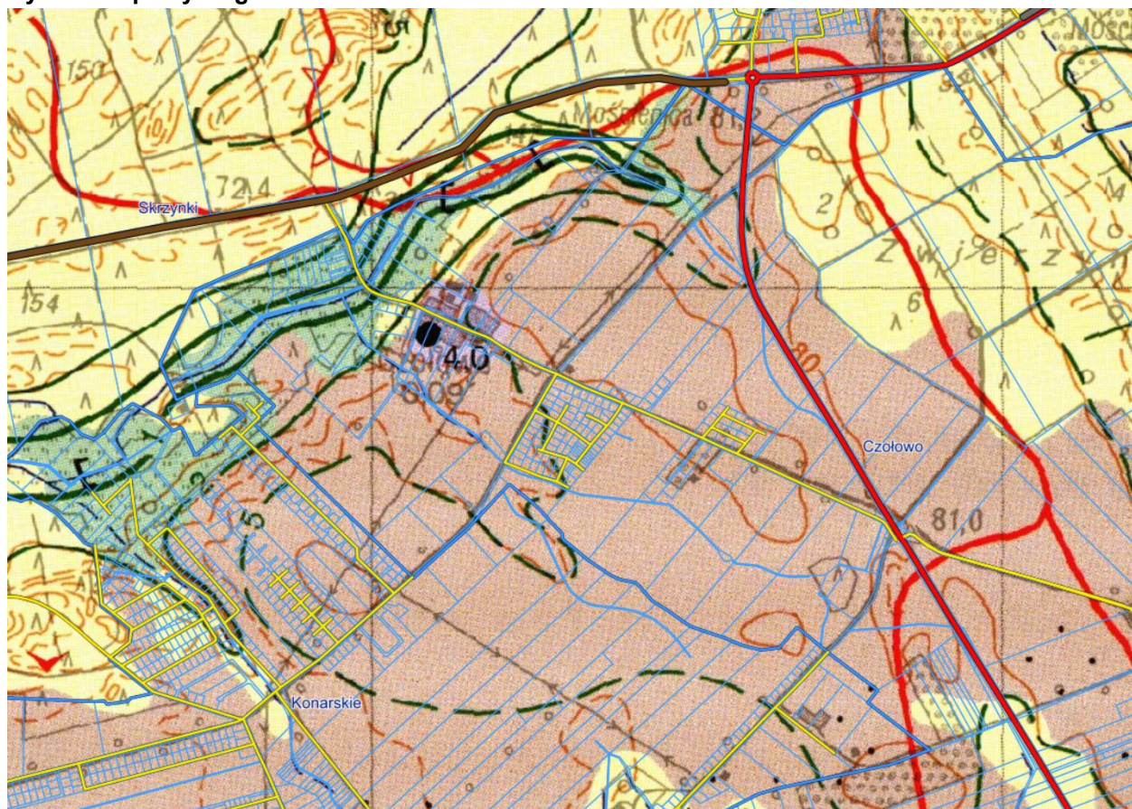
Ryc. 18 Mapa hydrograficzna
