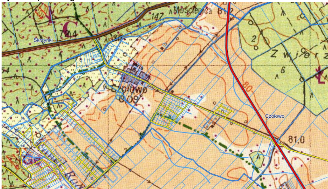
Ryc. 19 Mapa sozologiczna
